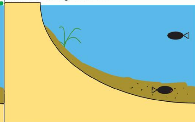
4. På grund av den höga nedbrytningen uppstår syrebrist vid botten, bottenlevande organismer dör
