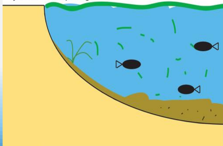
3. Vid algbloomningens slut faller alger ner till botten av sjön där nedbrytningen ökar
