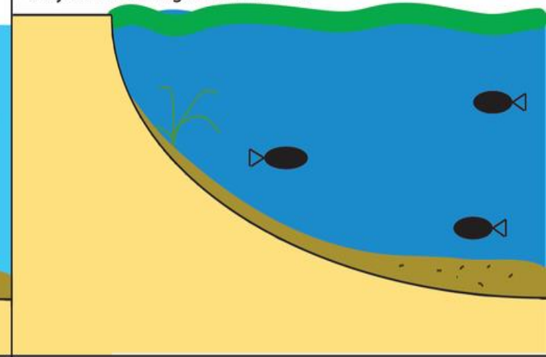
2. Sjö under algbloomning. Algerna bildar ett täcke som förhindrar solljuset att tränga mer i vattnet
